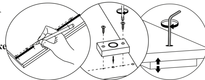
Рис. 3. Установка Опор
